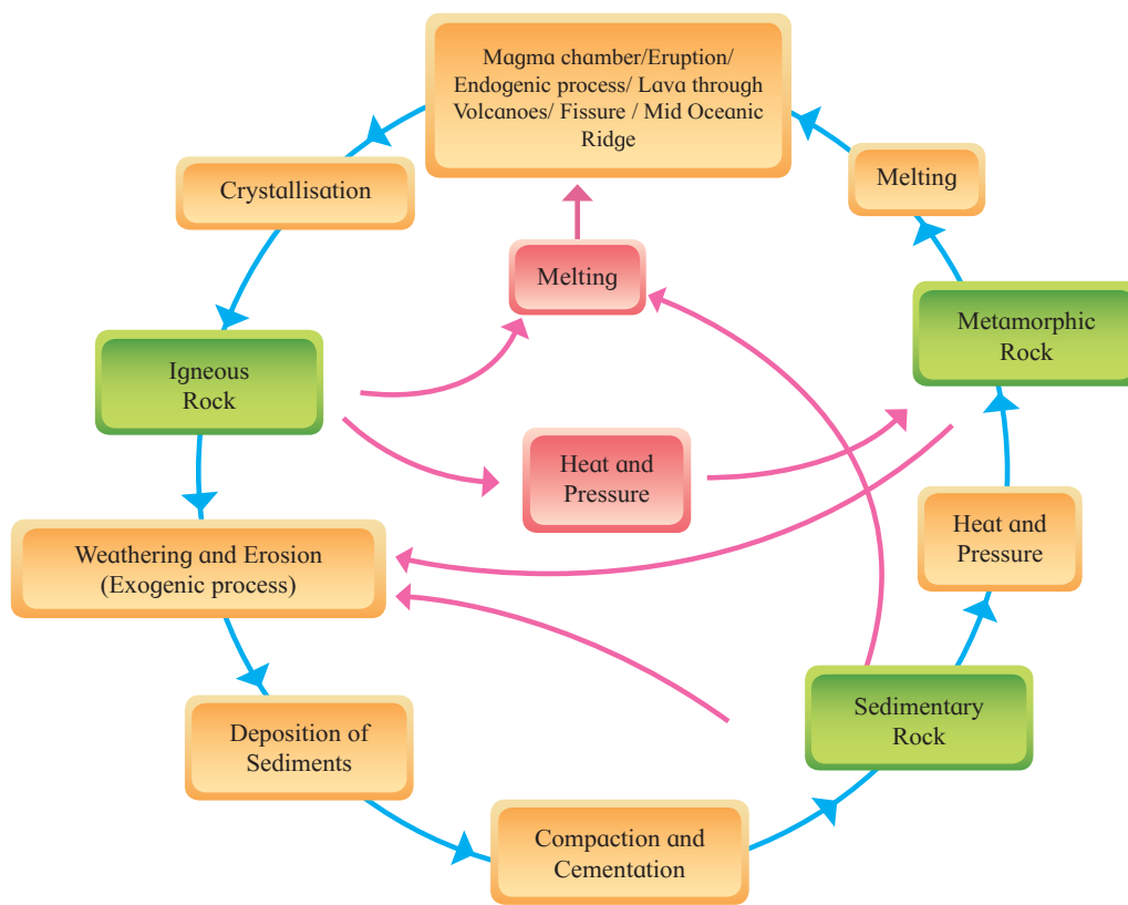
Fig. 4.1 : Rock cycle
